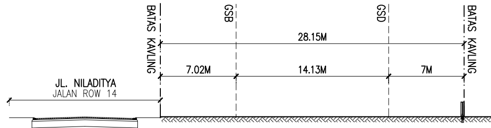
POT. A MEMANJANG KAVLING SKALA 1 : 350
